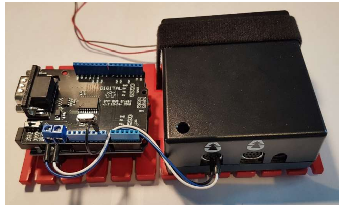
De werkende testopstelling:
